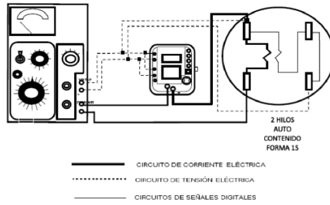
Figura 5.4-Conexión con carga artificial sistema 1 fases 2 hilos con medidor autocontenido.
